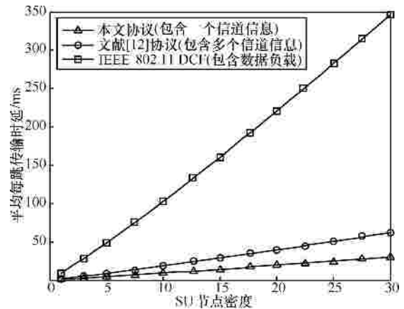
(b) 满负载时平均每跳时延比较
