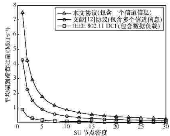
(a) 满负载时平均端到端吞吐量比较
