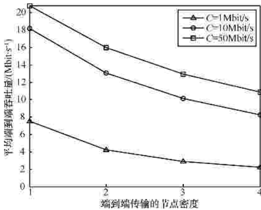
(a) 空负载时平均端到端吞吐量比较
